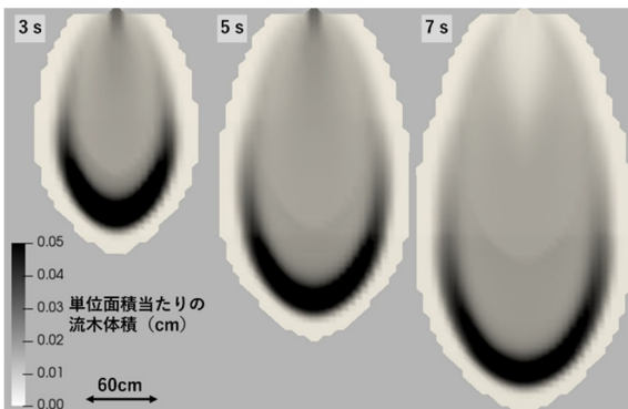
図-5. 流木輸送濃度式を導入した場合の計算結果
