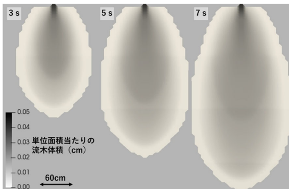
図-4. 流木輸送濃度式を導入しない場合の計算結果
